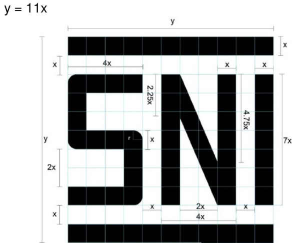
Gambar 2. Ukuran Tanda SPPT SNI
